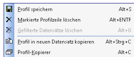
Abb. 9.60 Das Profilzeilen-Kurzmenü
