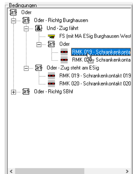
Abb. 12.10 Einträge verschieben
