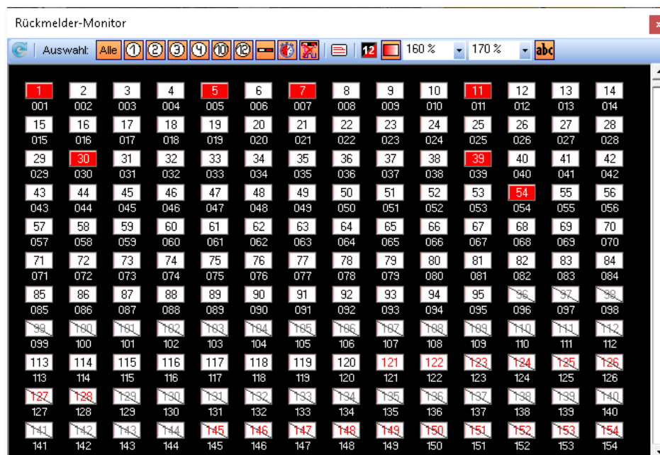
Abb. 16.97 Der Rückmelder-Monitor
