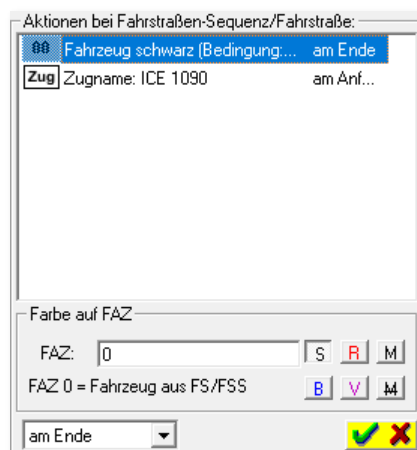
Abb. 10.37 Zwei Schaltaktionen
