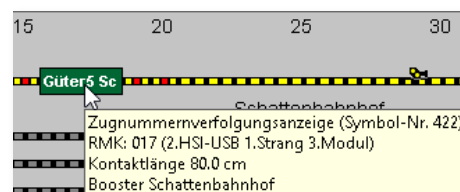
Abb. 16.48 Zugnummernverfolgungsanzeige belegt
