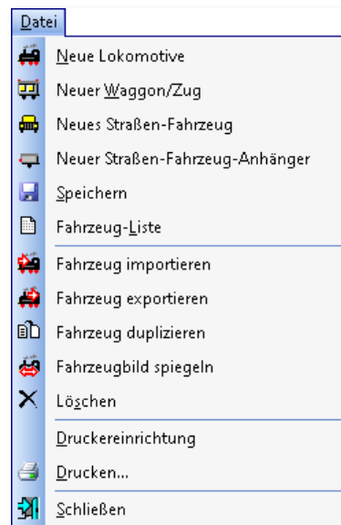
Abb. 4.67 Die Druckfunktion
