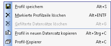
Abb. 9.58 Das Profilzeilen-Kurzmenü
